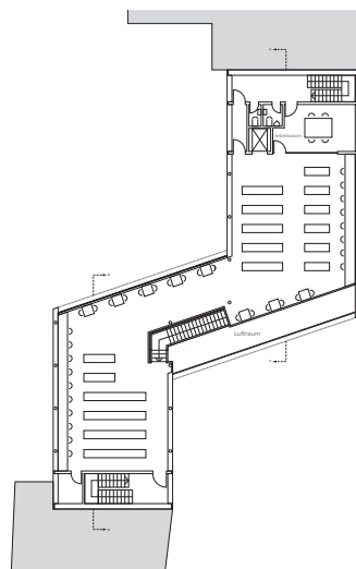
Grundriss_2. OG
