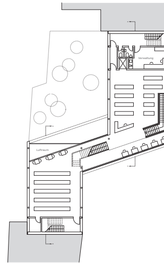
Grundriss_1. OG
